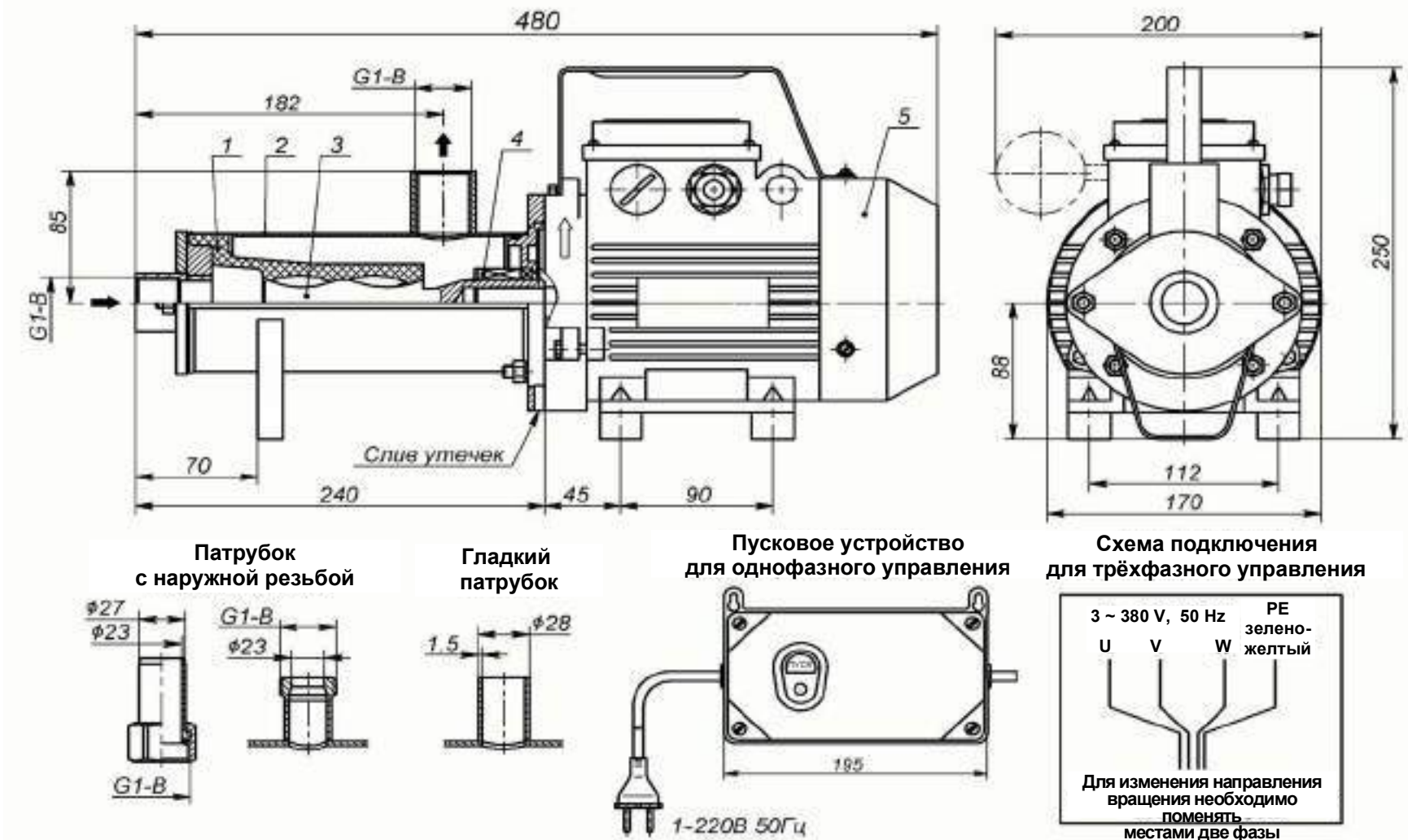
Рисунок 3 – Устройство насосов БУРУН СХ: 0,9/4-0,25/8, 1,2/4-0,37/6, 1,8/4-0,55/4, 3,6/4-0,75/2.
