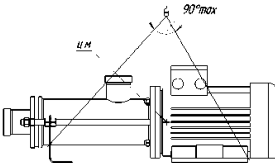
Рисунок 7 – Схема строповки
