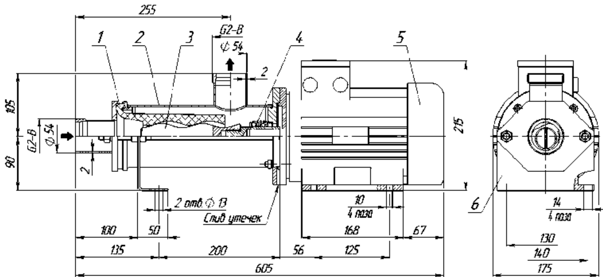
Рисунок 2 – Устройство насоса БУРУН СХ 6/4 – 1,5/4.
