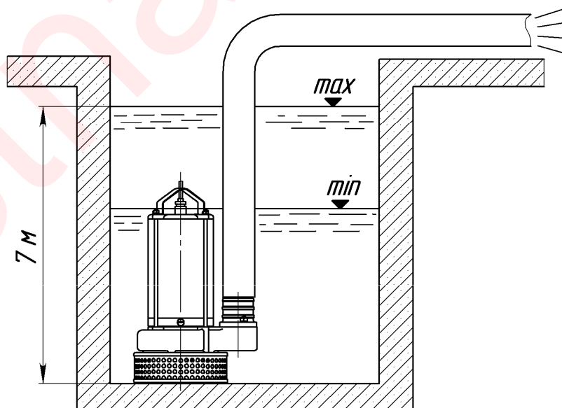
Рисунок 6 - Схема установки насоса Гном
