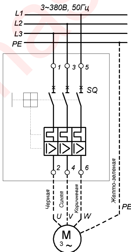
Рисунок 5 – Схема подключения насоса Гном
